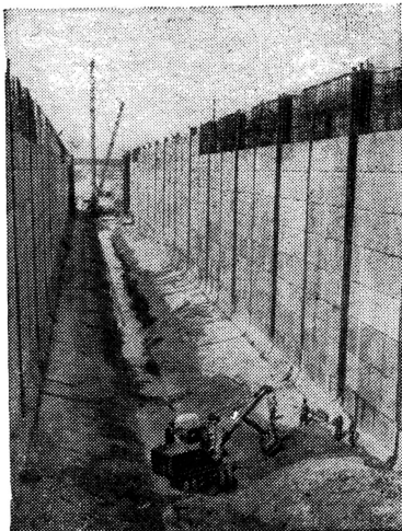
Вид камеры шлюза № 1 со стороны верхнего бьефа.
