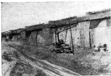
Эти бетонные стены — «берега» будущего шлюза.
